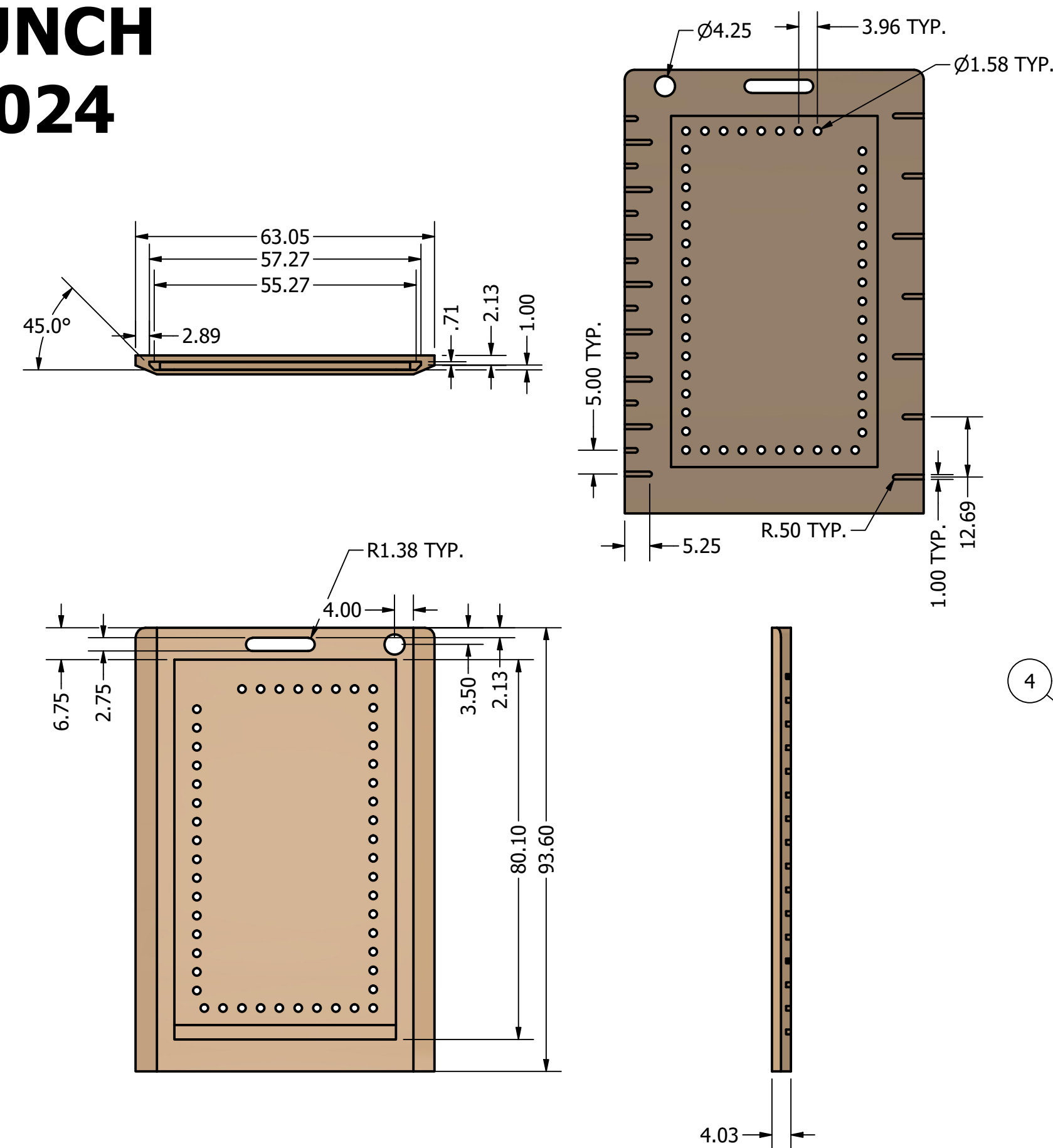
ID BODY SCALE 1:1
