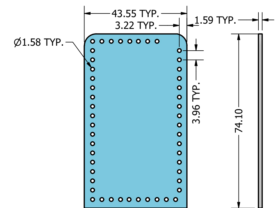
WALLET LAYER 1 SCALE 1:1
