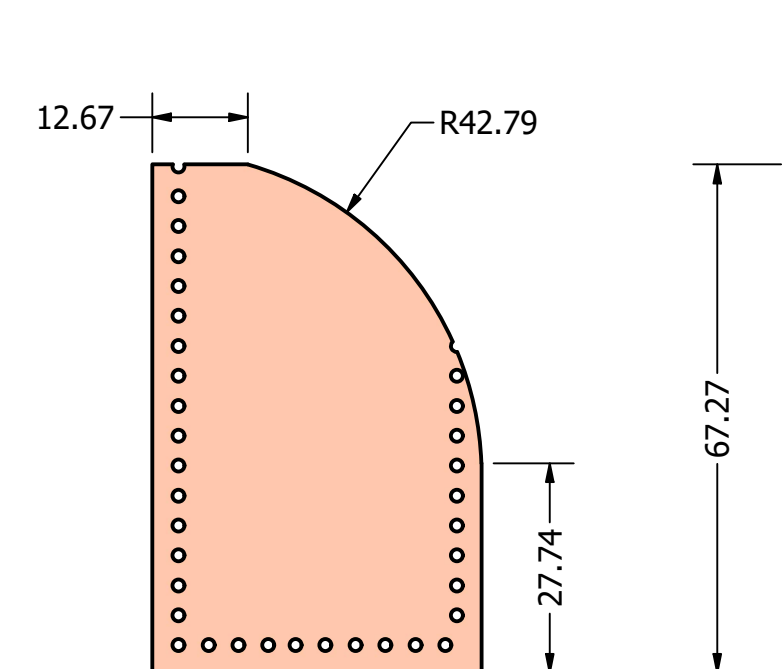
WALLET LAYER 2 SCALE 1:1
