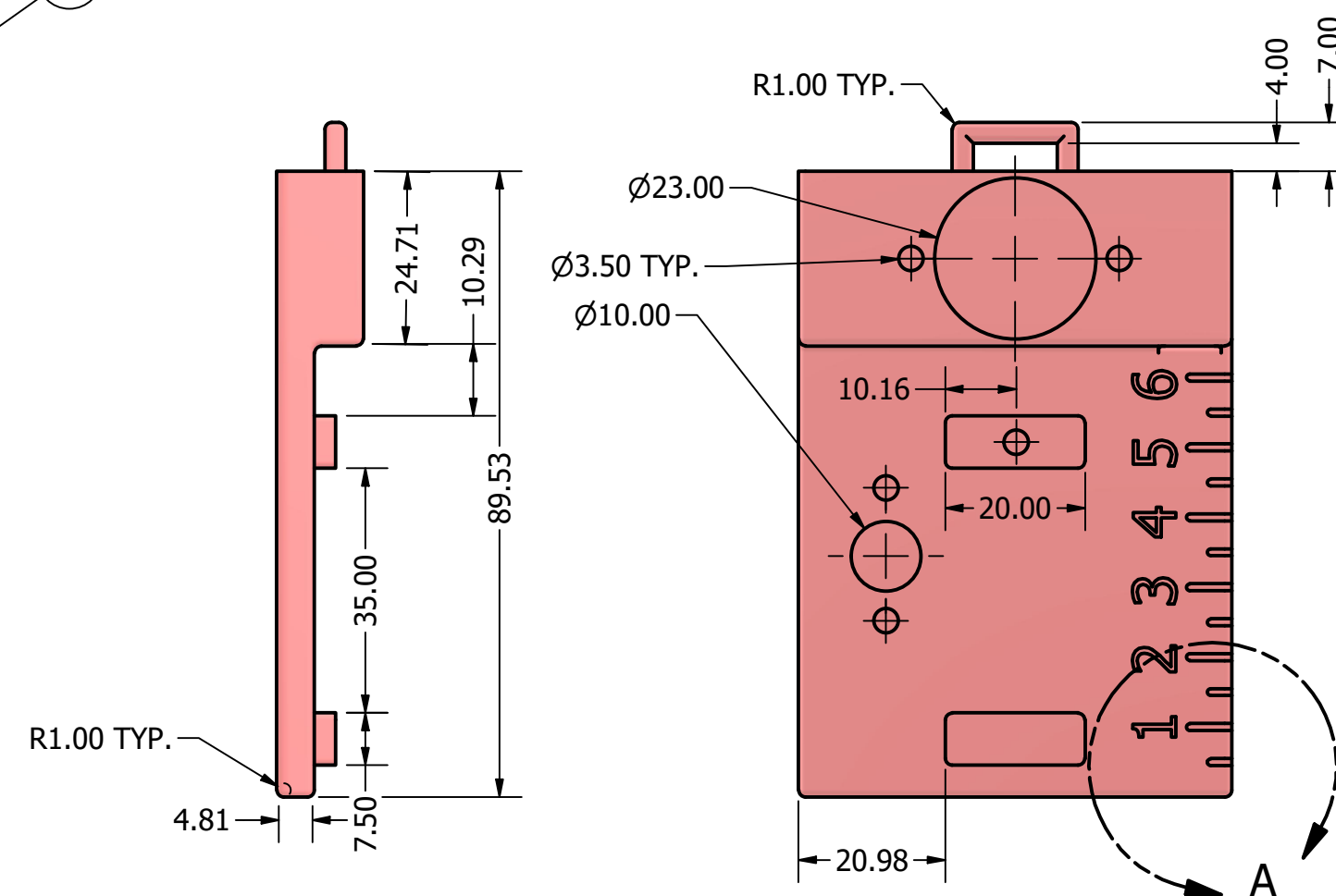
ID BODY SCALE 1:1
